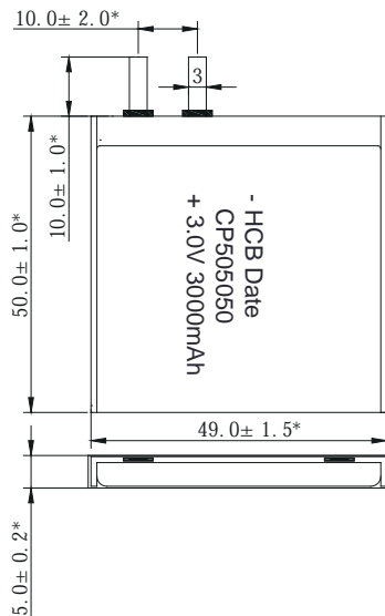
Dimensions in mm (GB1804-m)
