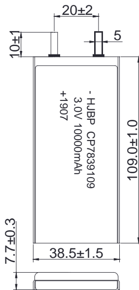
Dimensions in mm (GB1804-m)
